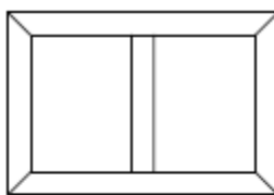
Размер для раскроя импоста = X + 8,5 мм
